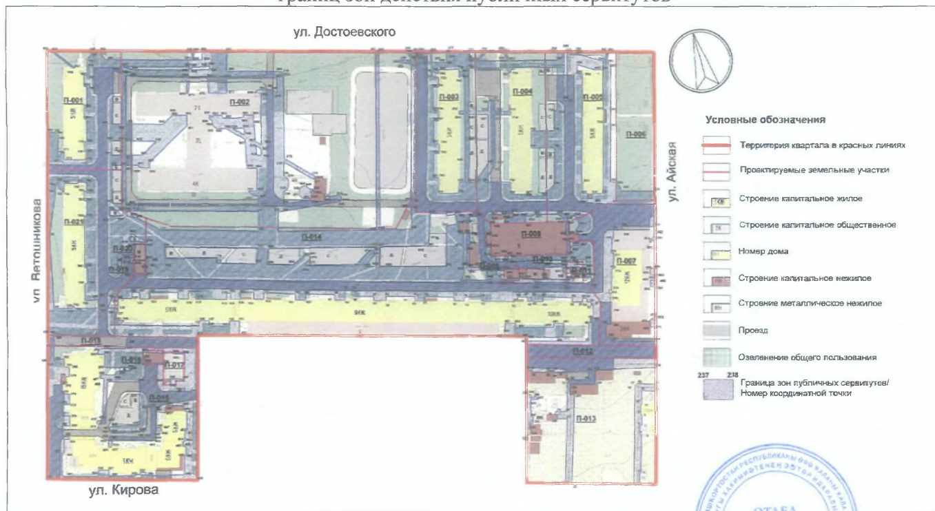
Чертеж межевания территории с отображением красных линий, линий регулирования застройки, границ зон действия публичных сервитутов
