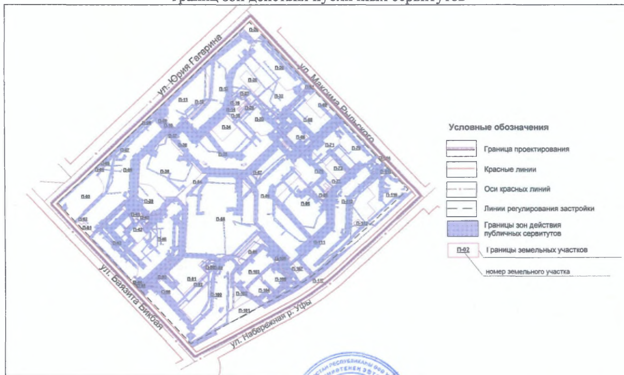
Чертеж межевания территории с отображением красных линий, линий регулирования застройки, границ зон действия публичных сервитутов
