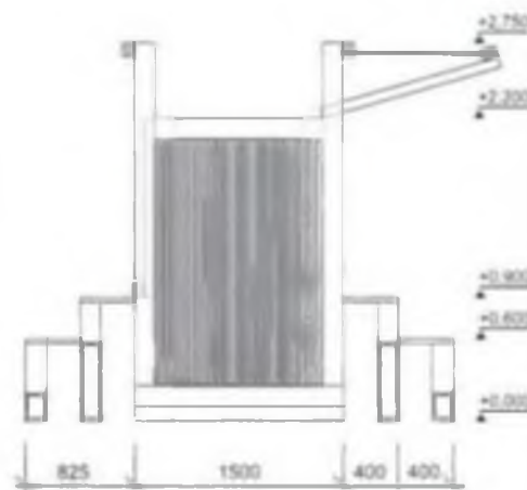
Фасад М 1:100
