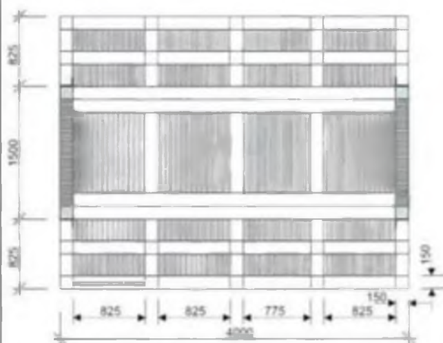
План М 1:100
