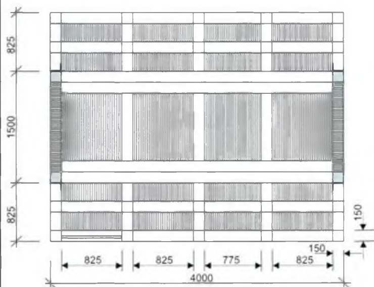
План М 1:100
