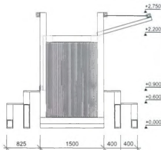
Фасад М 1:100
